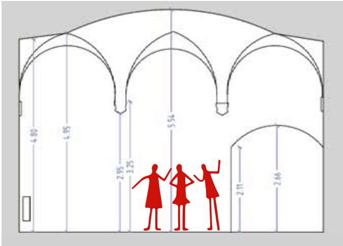
sezione A-A
